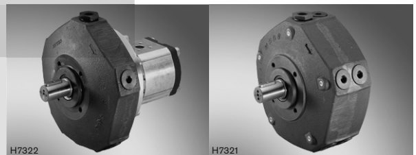
H7322 P2R4-3X/4,00-700RK01M01+AZPF8
