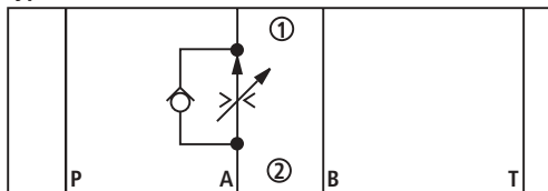
Type Z2FRM 6 A...
