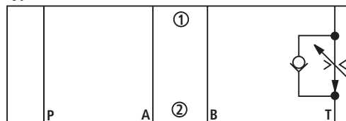
Type Z2FRM 6 T...
