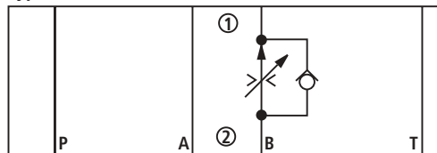
Type Z2FRM 6 B...
