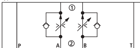
Type Z2FRM 6 C...
